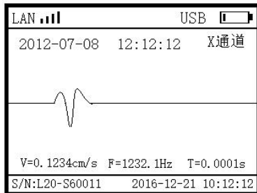
波形预览
