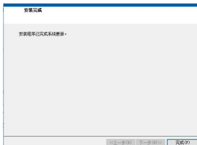
安装完成
