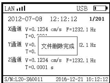
文件删除
