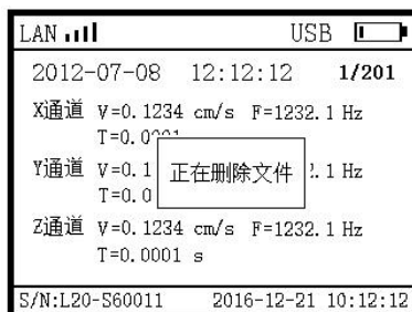
正在删除
