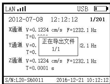
正在导出
