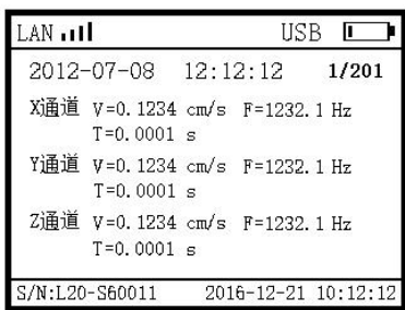
返回特征值
