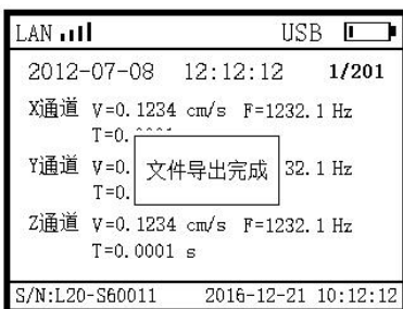
文件导出
