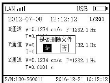
删除指令
