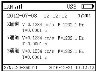
幅值预览
