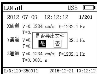
导出指令
